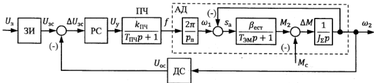
Рисунок 8 - Структурная схема замкнутой по скорости системы скалярного управления: ЗИ - задатчик интенсивности; РС - регулятор скорости; ПЧ - преобразователь частоты; АД - асинхронный двигатель с короткозамкнутым ротором; ДС - датчик скорости
