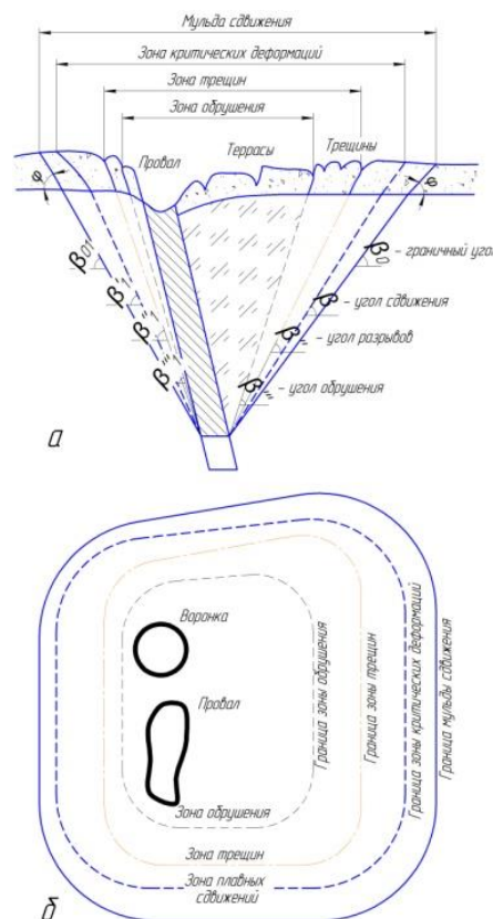
Рис. 1.1. Формы проявления процесса сдвижения: а – на разрезе вкрест простирания рудного тела; б – на плане земной поверхности
