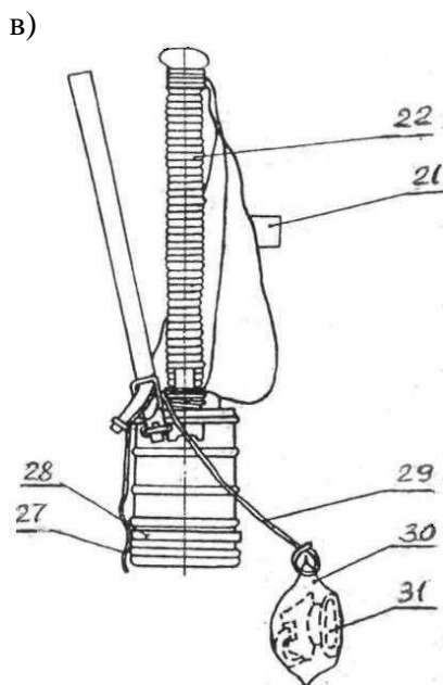
Рис. 1.2. Изолирующий самоспасатель ШСС-Т
