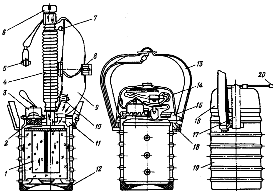
Рис. 1.1. Изолирующий самоспасатель ШСС-1
